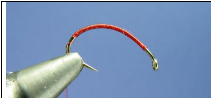
ETAPE 1 : Placez dans votre étau un hameçon caddis n°14 et faites un enroulement de fil de montage rouge.
