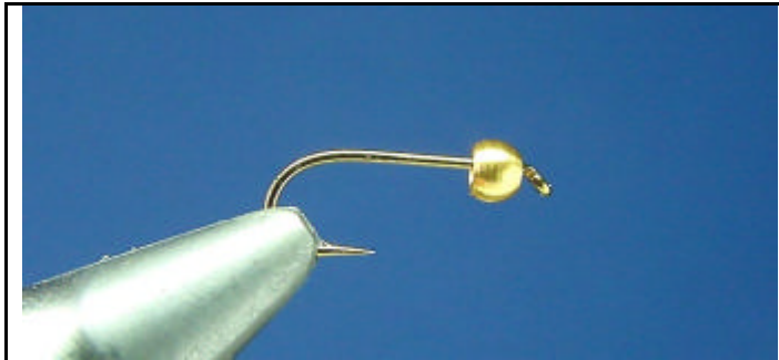
ETAPE 1 : Placez dans votre étau un Hameçon n°16 avec une bille nympe or 2mm.
