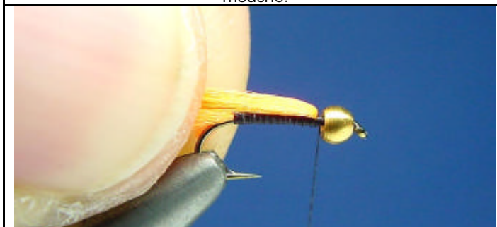
ETAPE 7 : Placez le fil de montage entre les brins de polyfloss et la bille.
